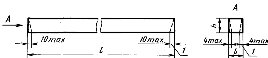
Перемычка типа ПБ
